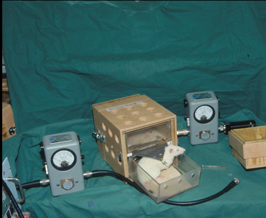
The TEM cell
